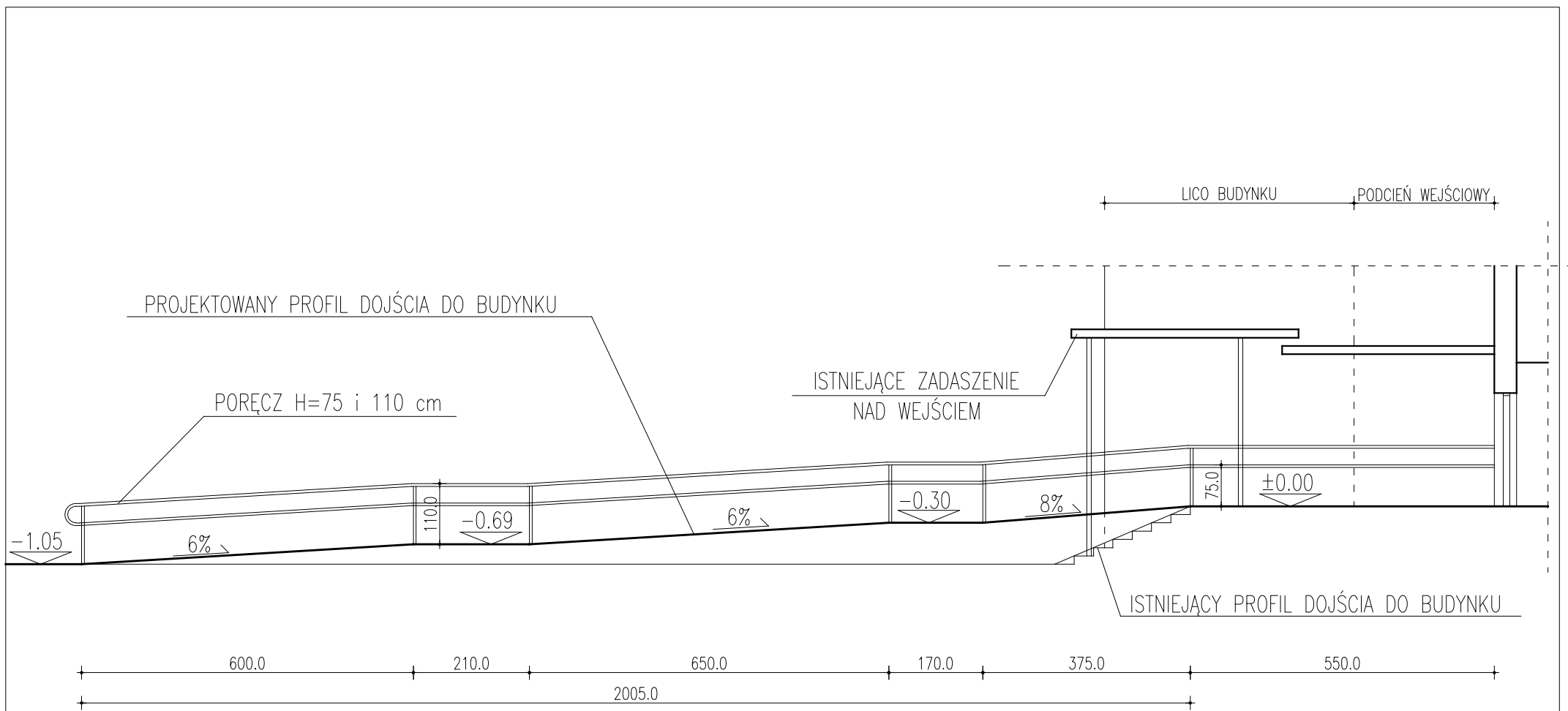
PROFIL TERENU SKALA 1:100
